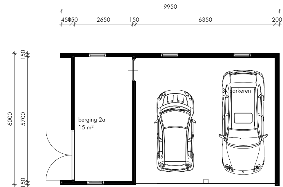
Begane Grond schaal 1:100
