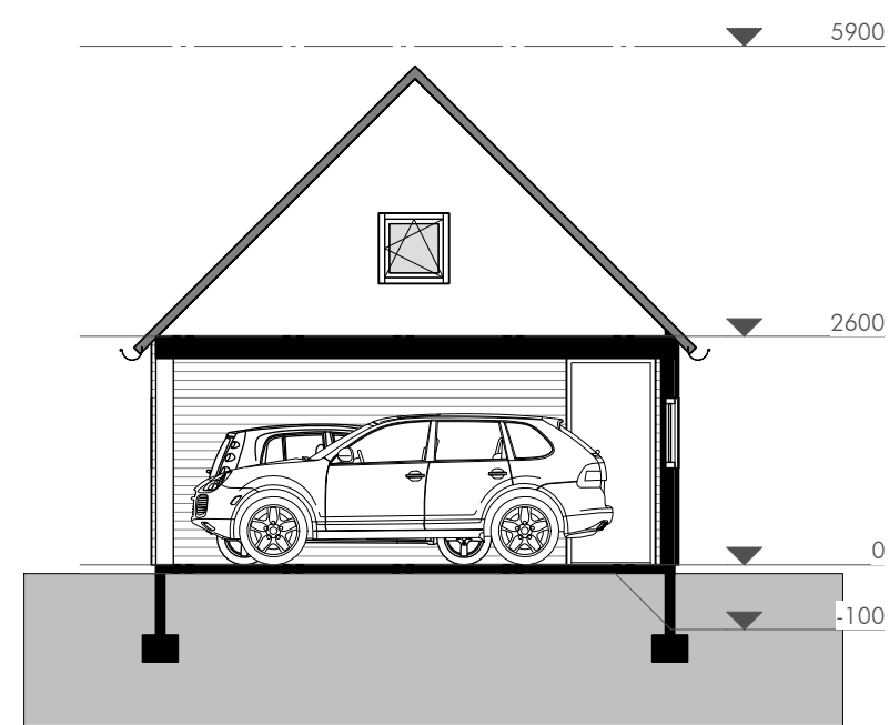
Doorsnede schaal 1:100
