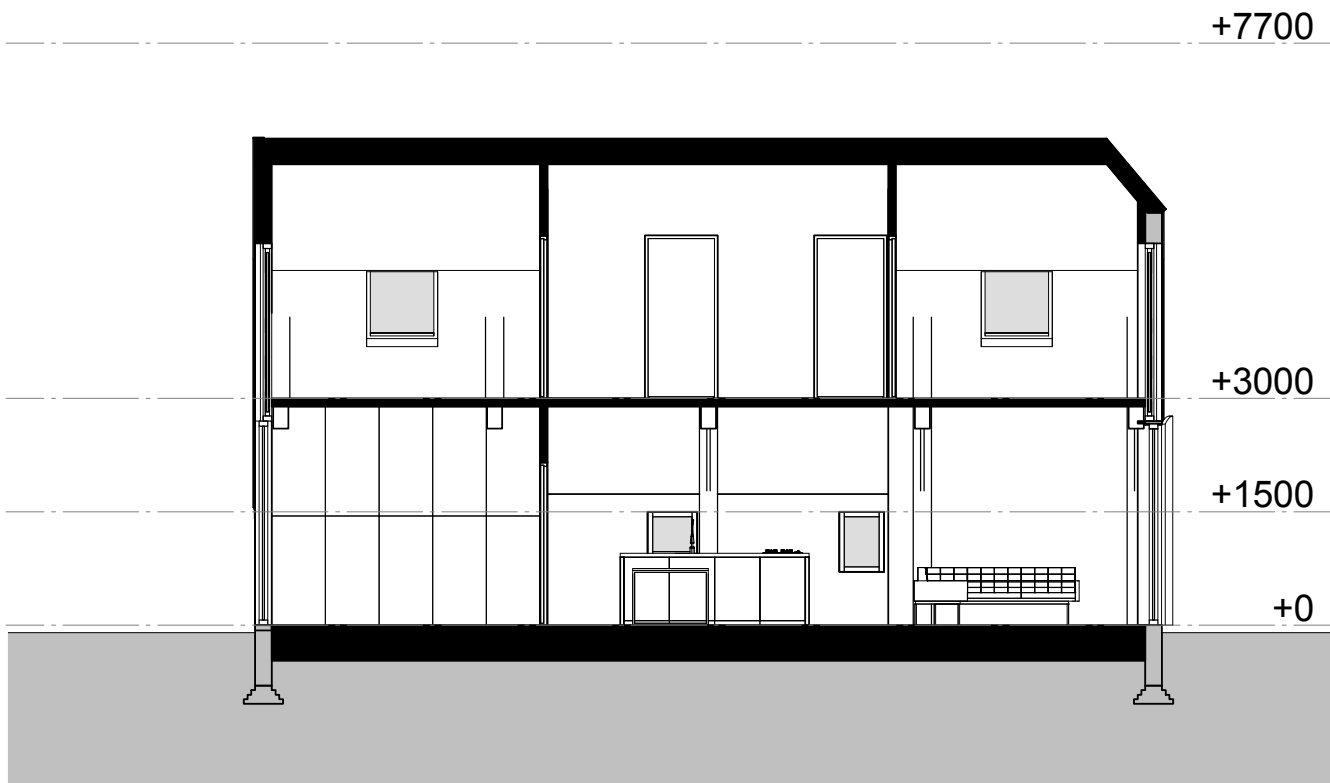
Doorsnedes schaal 1:100
