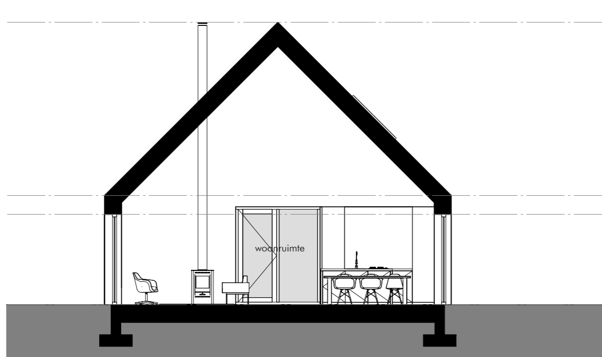
Doorsnedes schaal 1:100
